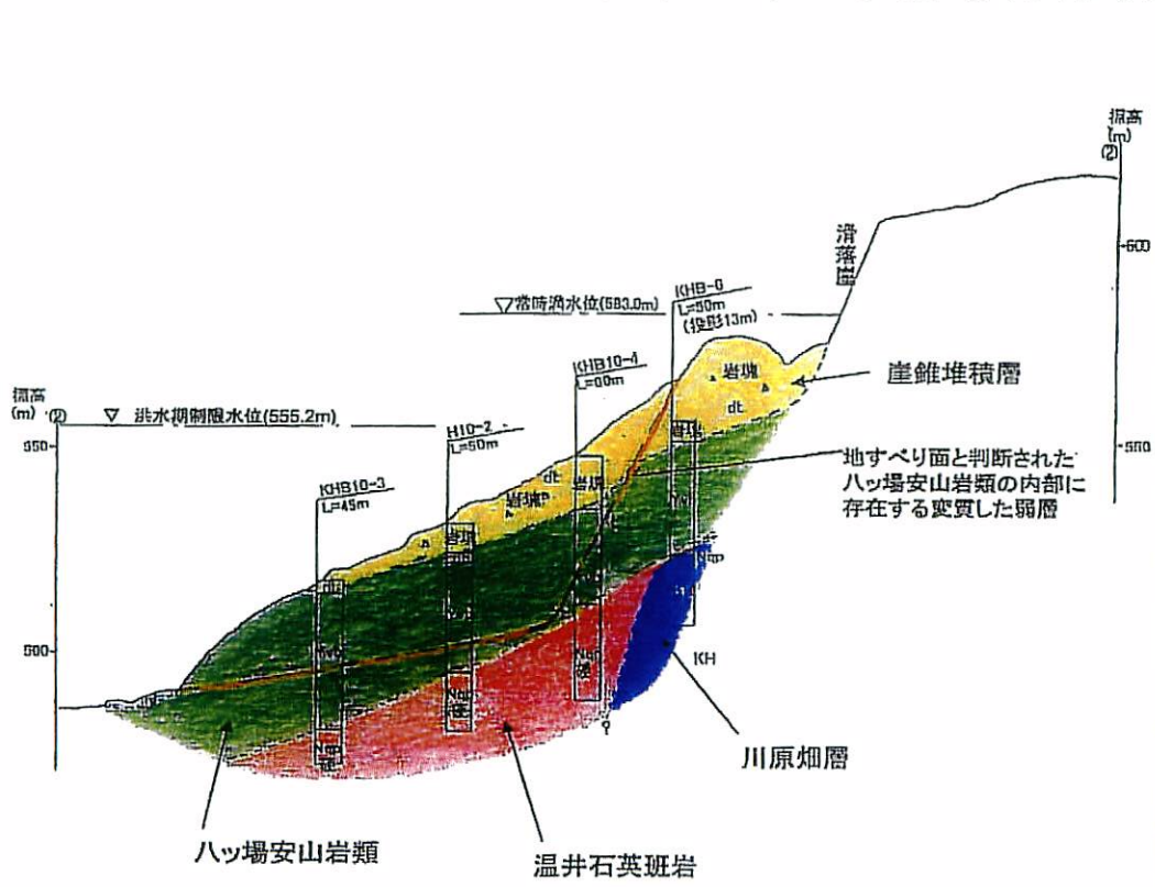
川原畑地区二社平 地すべり断面図及び状況写真
