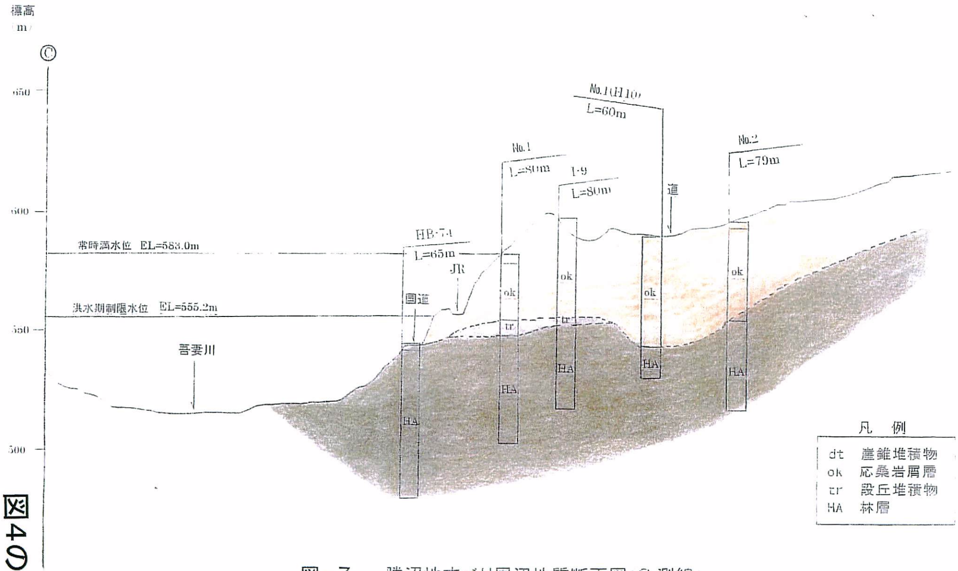
図-7 勝沼地すべり周辺地質断面図(C測線)
