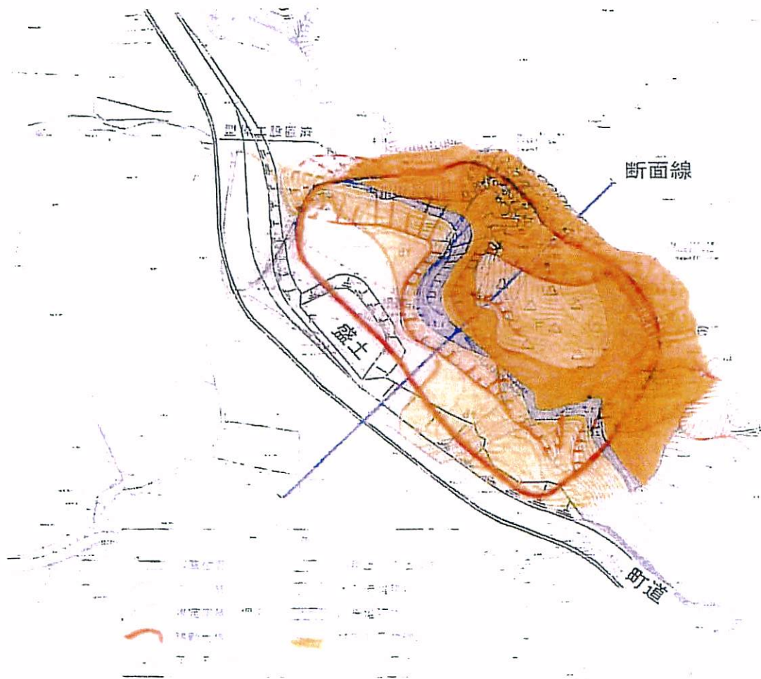
図-12 横壁小倉地区平面図
