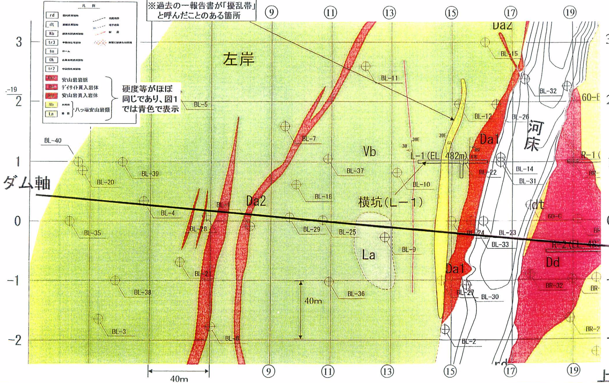
図4-7 左岸地質断面図(標高480m断面の平面図)(乙172-2・図8より)
