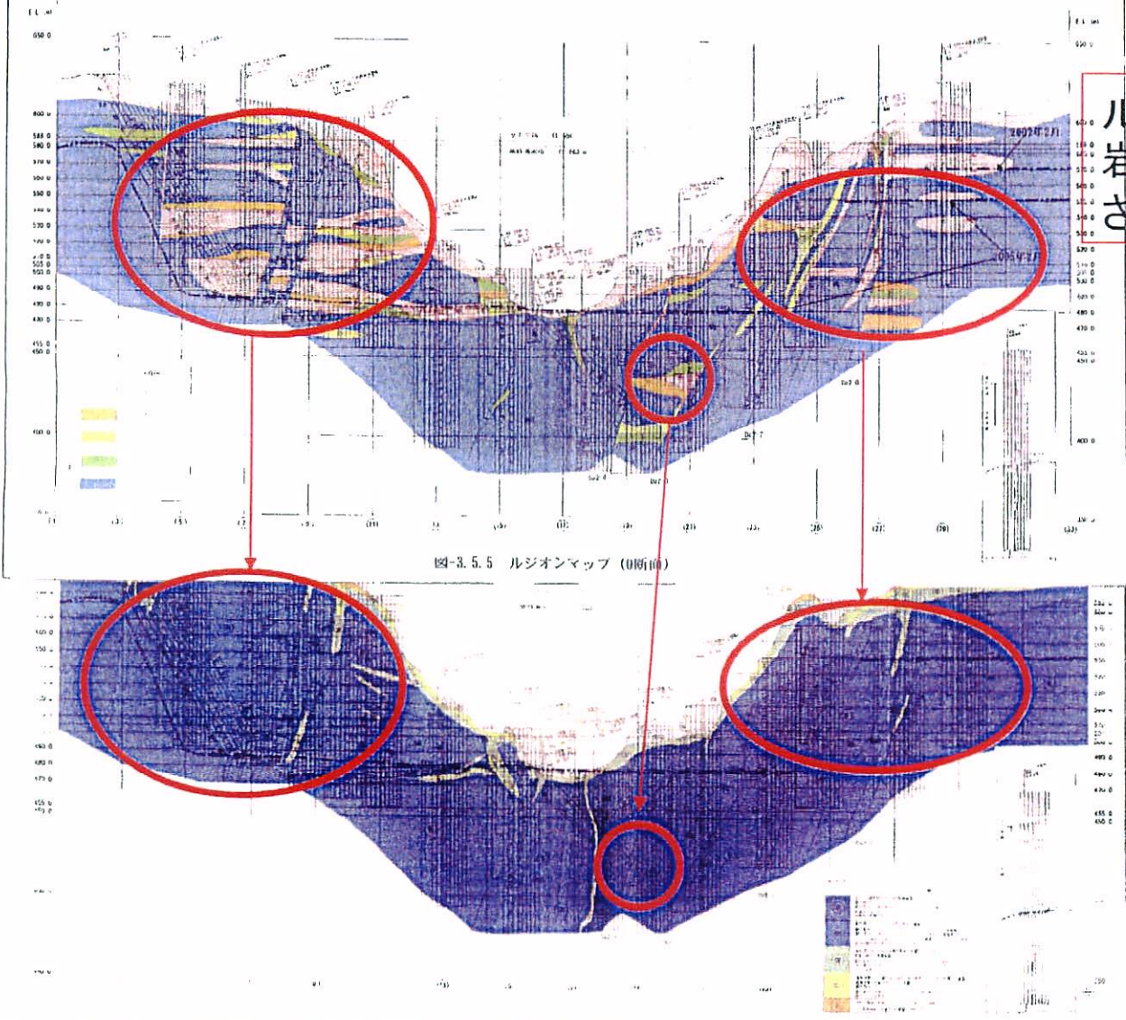
図-2 ルジオンマップ(上)と岩級区分図(下)の対比(0測線)
