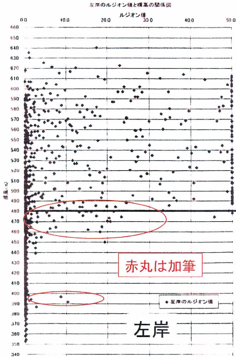
図-7.6.2 左岸のルジオン値と標高の関係図
