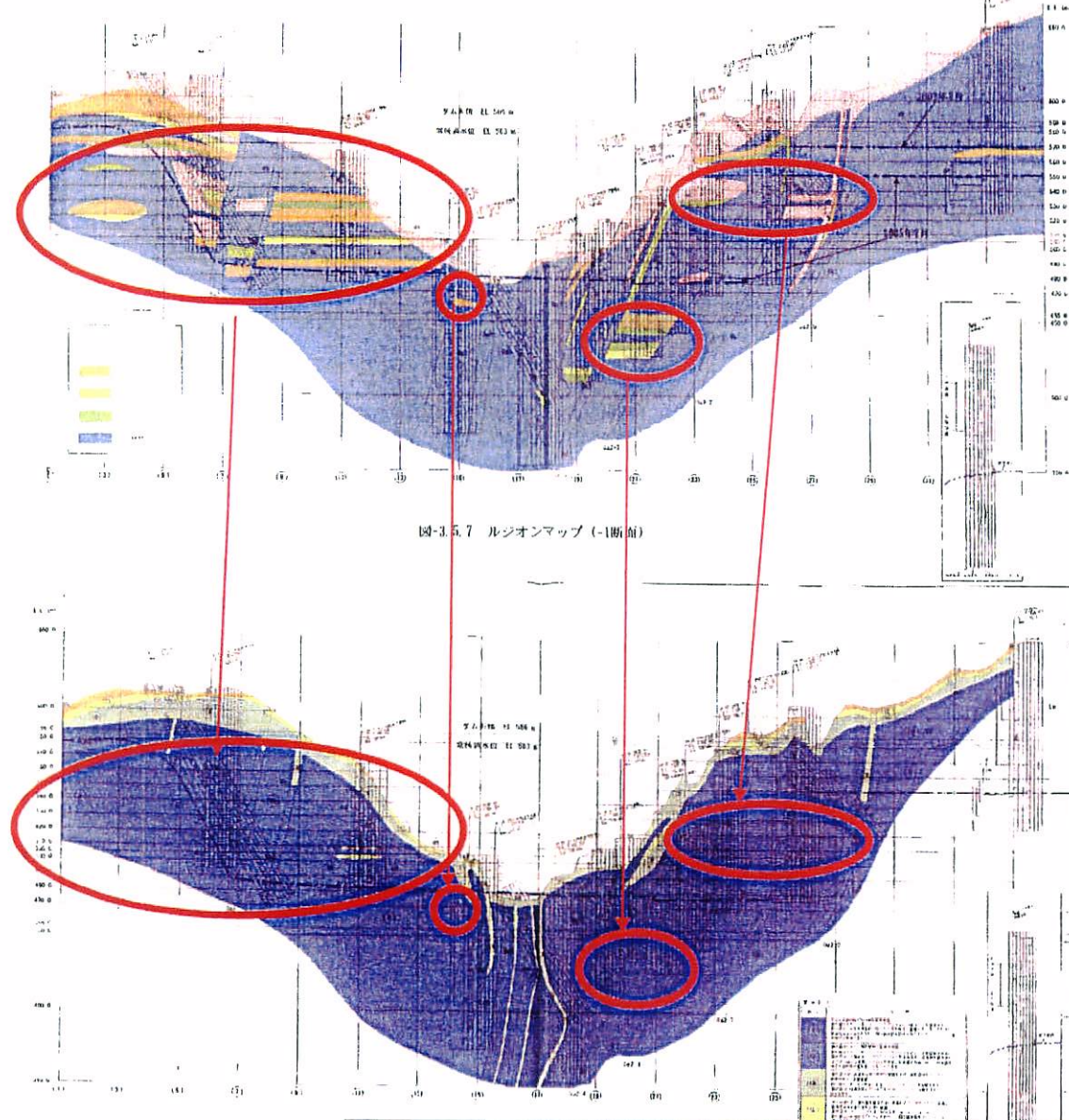
図-1 ルジオンマップ(上)と岩級区分図(下)の対比(-1測線)
