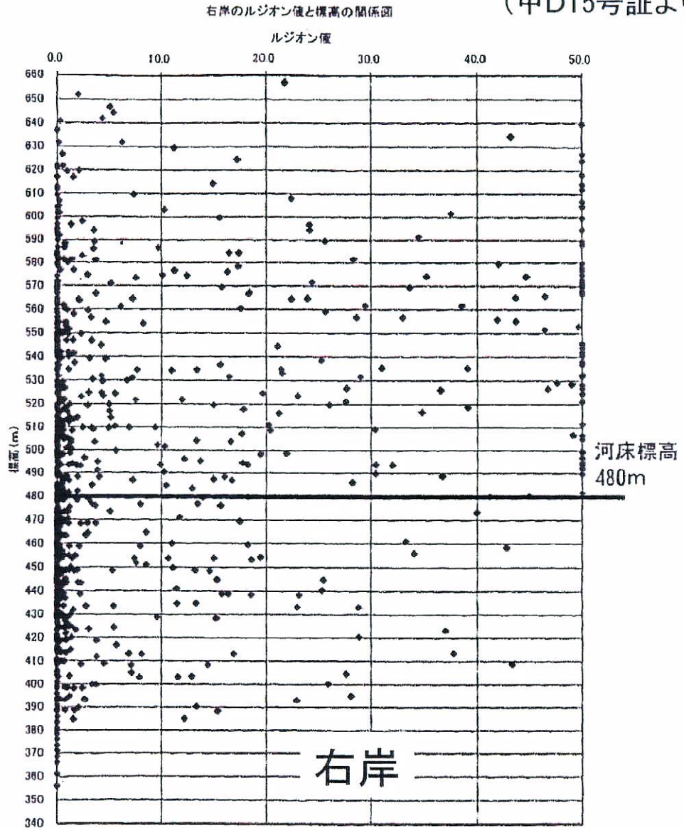
図-7.8.2 右岸のルジオン値と標高の関係図
