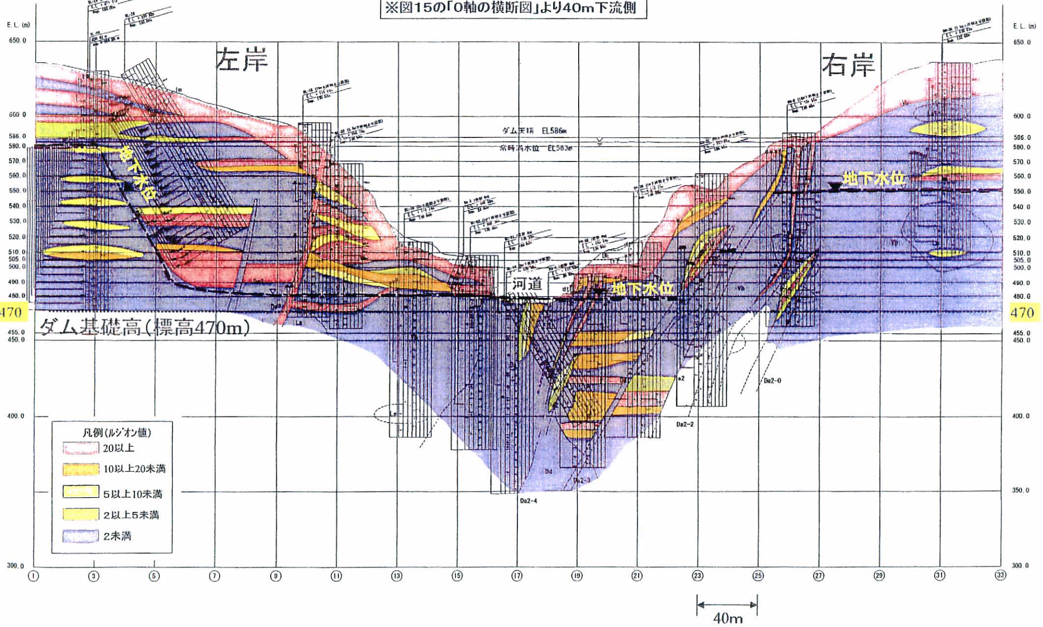
図4-10 ルジオンマップ(1軸の横断図)(乙172-2・図16より)
