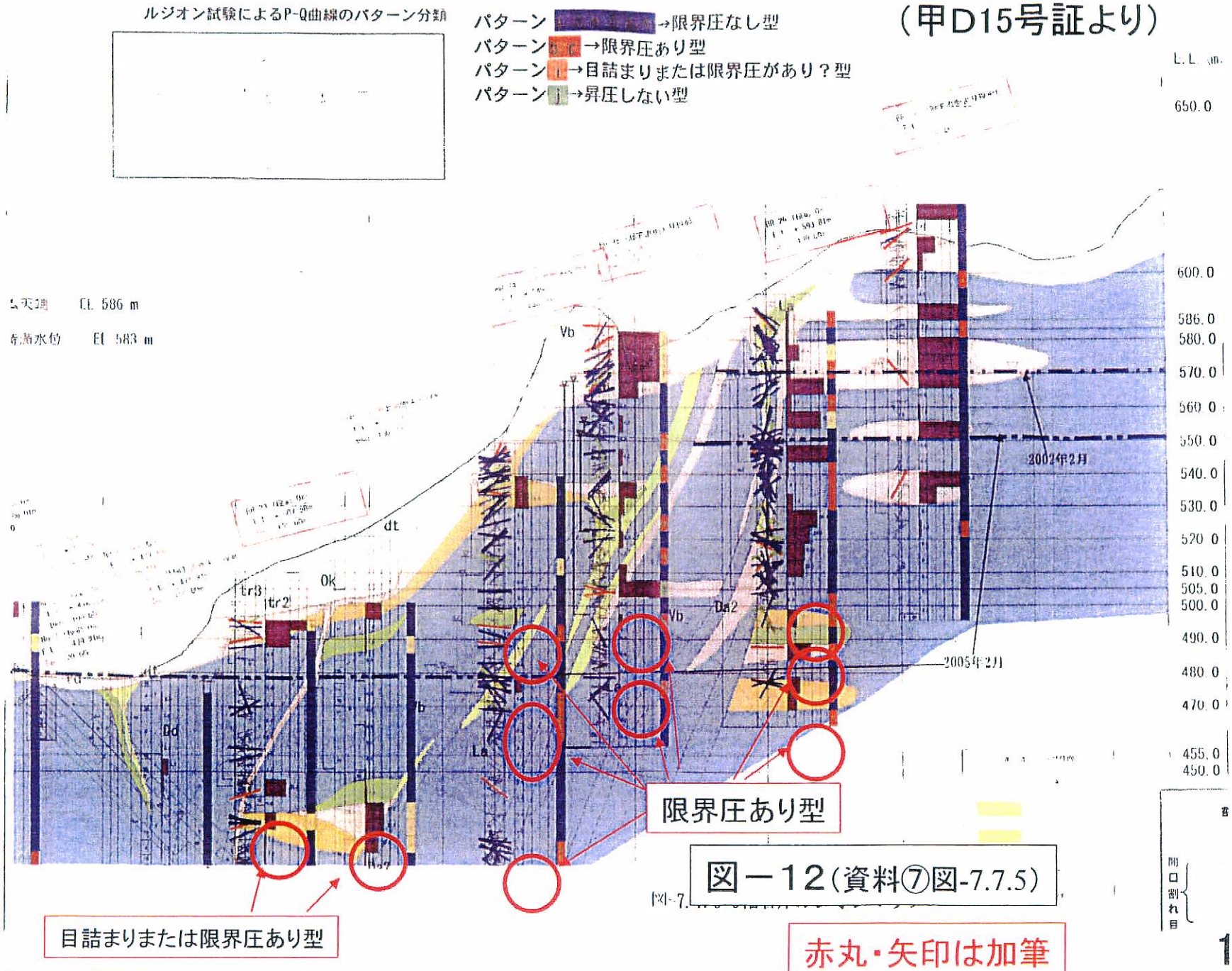
図4-13 ルジオンマップとP-Q曲線のパターン(0軸右岸部)(甲D15・図12より)
