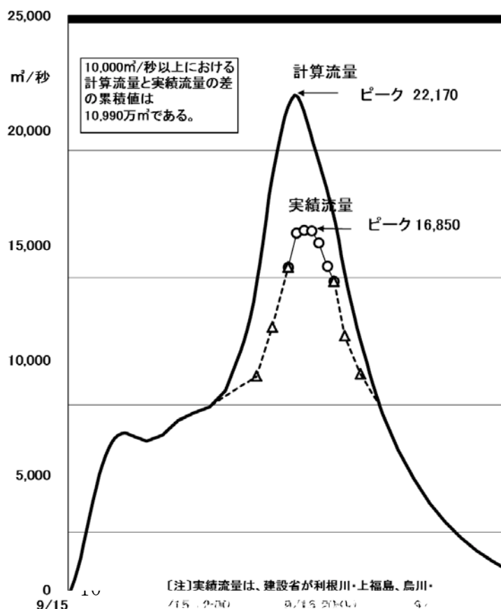
国交省による1947年洪水の計算流量と実績流量（八斗島地点）
